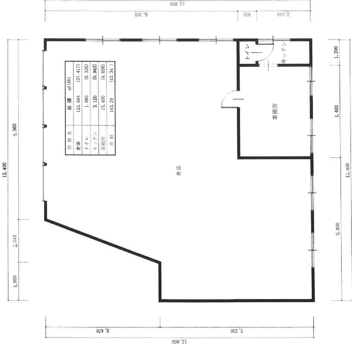
コーポ竹岡第2 1F 倉庫部分 平面図 S:1/100
